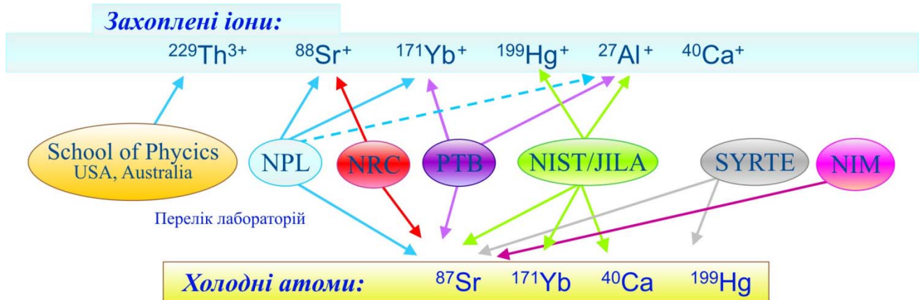
Рис. 2. Варіанти реалізації стандарту частоти оптичного діапазону
