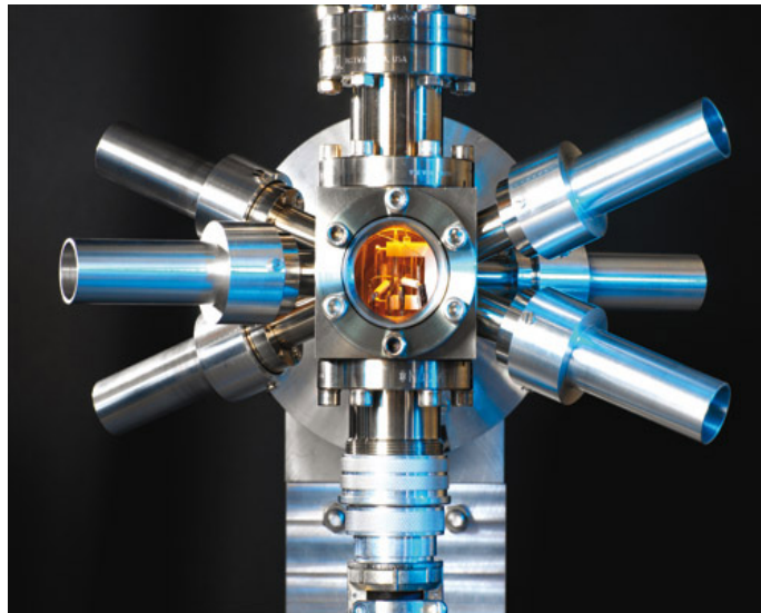
Рис. 1. Оптичний годинник на іонах стронцію
