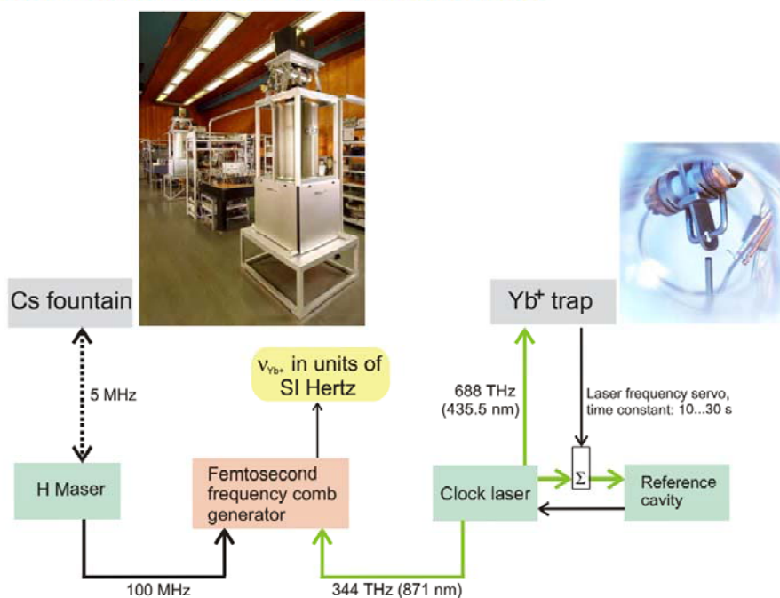
Рис. 3. Принцип побудови квантового генератора і вимірювання частоти оптичного діапазону
